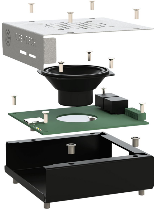
Demontaj
